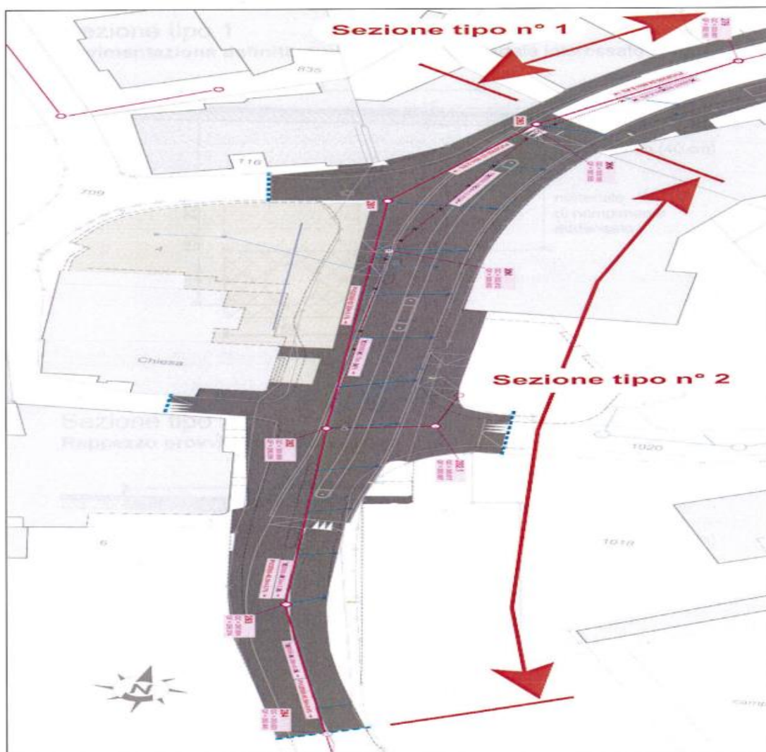
Estratto planimetria di progetto con le 2 sezioni tipo
